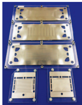
開発品「燃料電池の金属セパレーター」
